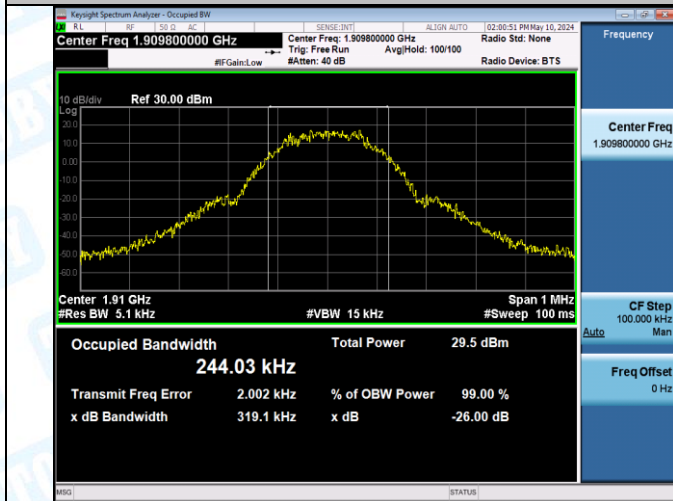
GPSS1900-810-0-PASS
