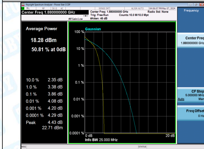
Band2-20MHz-QPSK-19100-1RB#0-PASS
