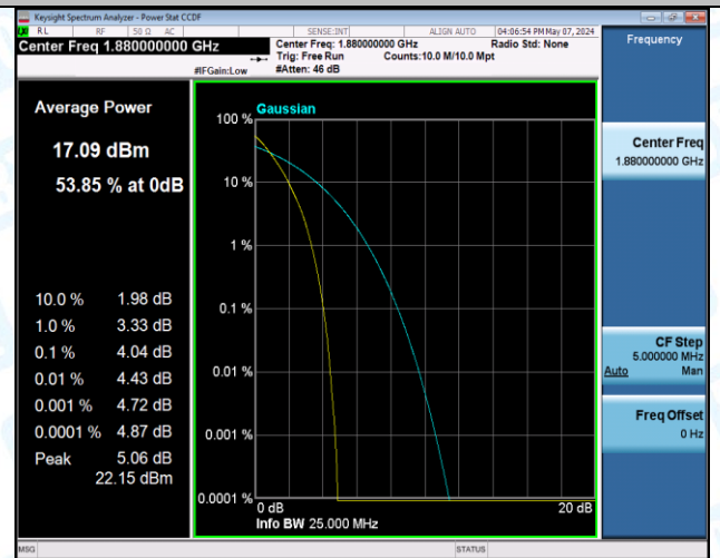
Band2-20MHz-QPSK-19100-100RB#0-PASS
