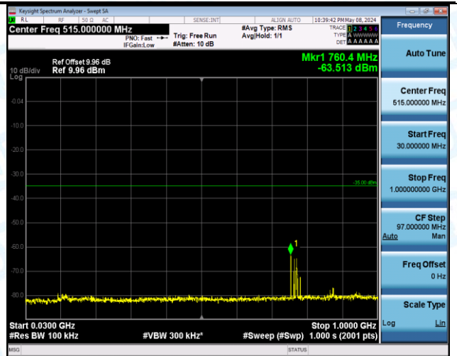
Band7_20MHz_QPSK_20850_1RB#99_20000~27000_20000~27000
