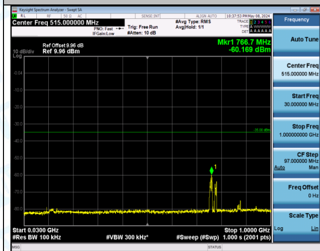
Band7_20MHz_QPSK_20850_1RB#0_20000~27000_20000~27000
