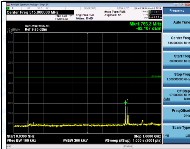
Band7_20MHz_QPSK_20850_100RB#0_20000~27000_20000~27000
