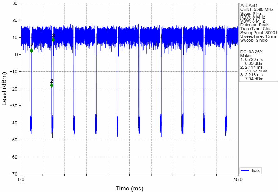
802.11a_MCH_5580MHz_Ant1_NTNV
