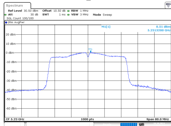
802.11n40_5230MHz
