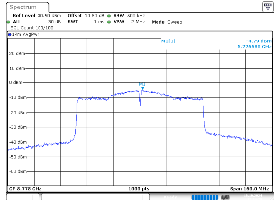
802.11ac80_5775MHz
