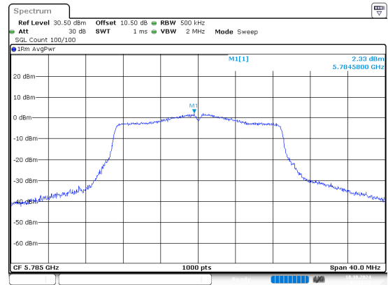
802.11n20_5785MHz
