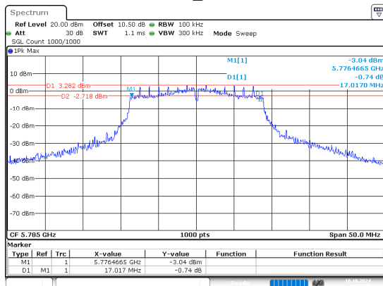
802.11n20_5785MHz
