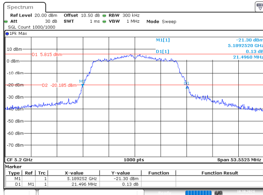
802.11n20_5200MHz
