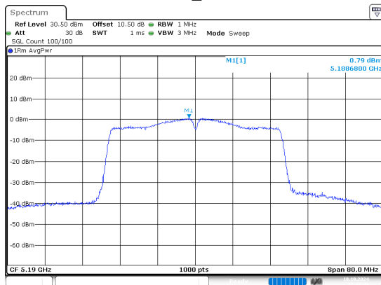
802.11n40_5190MHz
