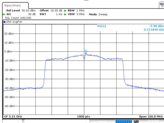
802.11ac80_5210MHz
