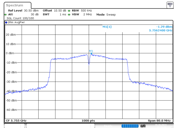
802.11n40_5755MHz
