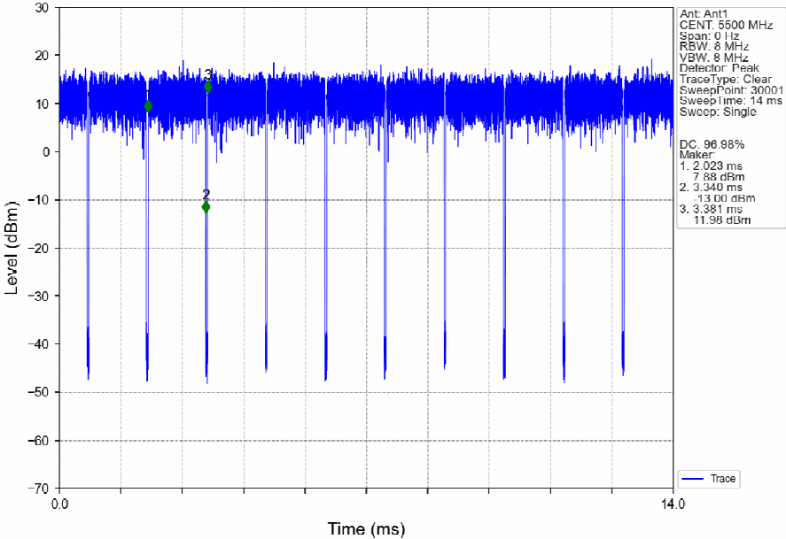
802.11ac(VHT20)_LCH_5500MHz_Ant1_NTNV
