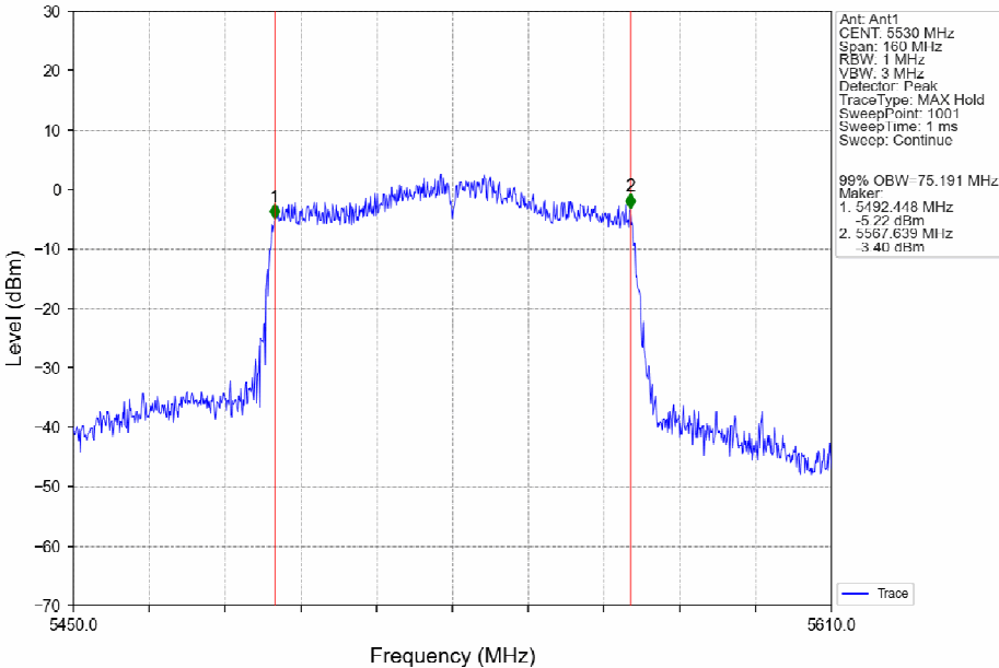
802.11ac(VHT80)_LCH_5530MHz_Ant1_NTNV
