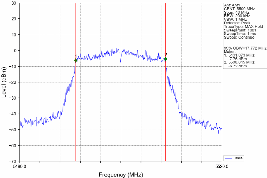
802.11ac(VHT20)_LCH_5500MHz_Ant1_NTNV
