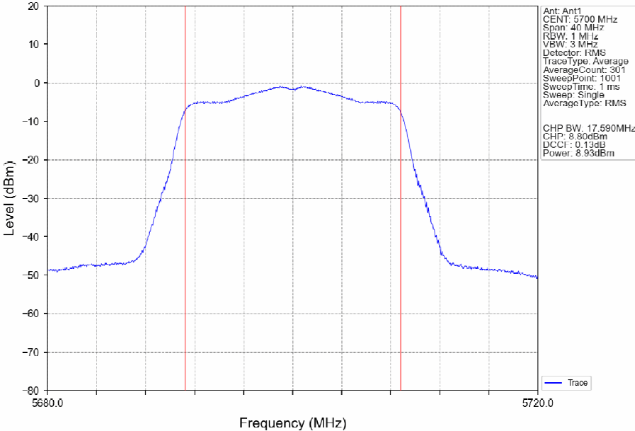
802.11ac(VHT20)_HCH_5700MHz_Ant1_NTNV
