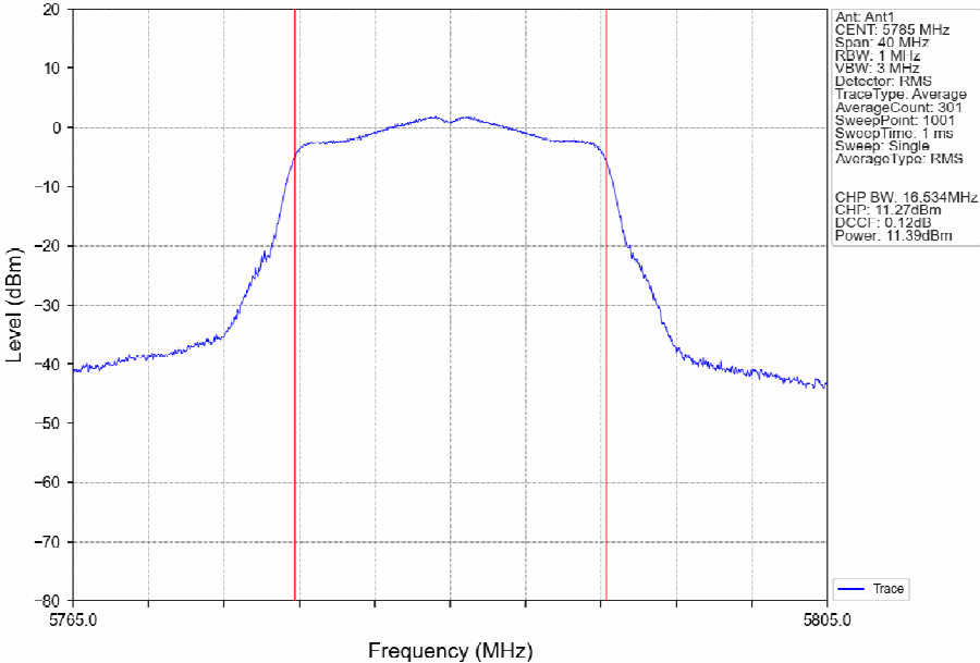
802.11a_MCH_5785MHz_Ant1_NTNV
