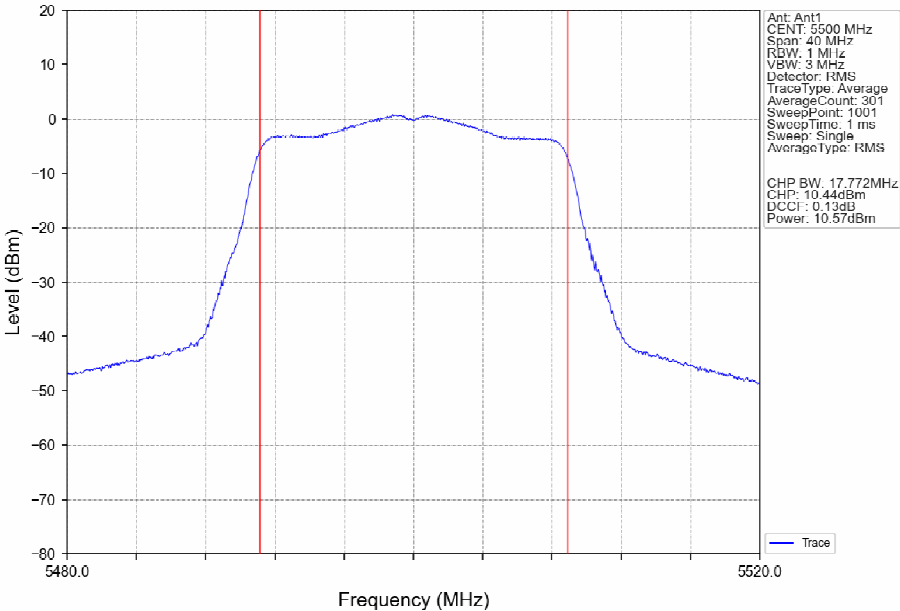
802.11ac(VHT20)_LCH_5500MHz_Ant1_NTNV
