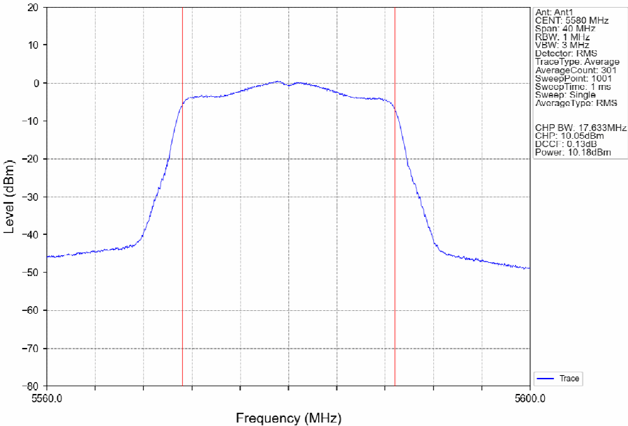
802.11n(HT20) MCH_5580MHz_Ant1_NTNV
