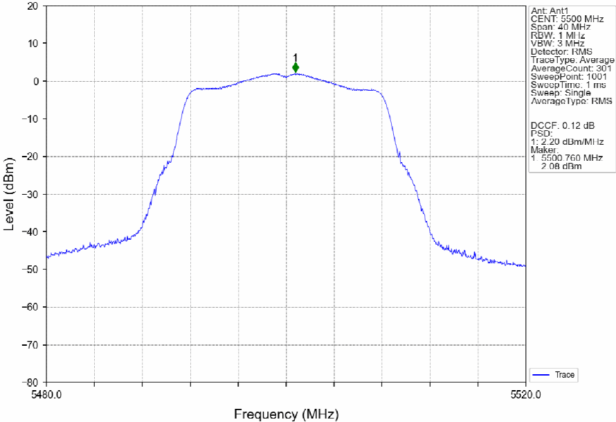
802.11a_LCH_5500MHz_Ant1_NTNV
