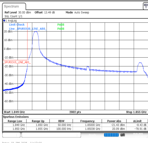
Band2-5MHz-16QAM-18625-1RB#0-PASS
