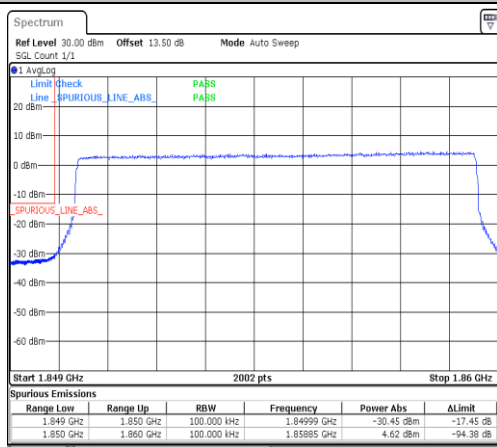
Band2-10MHz-QPSK-18650-1RB#0-PASS
