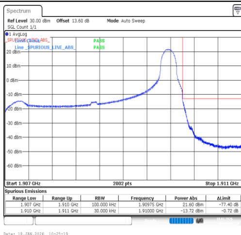
Band2-3MHz-QPSK-19185-1RB#14-PASS
