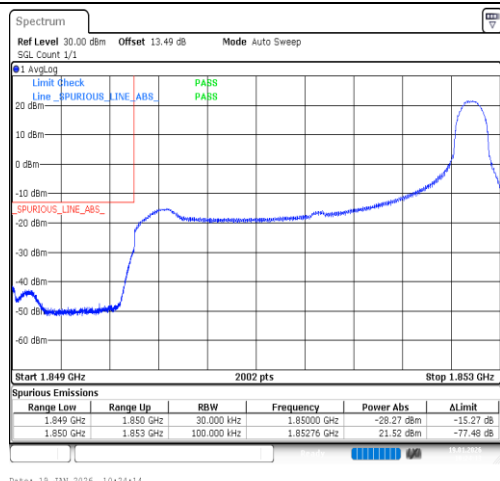
Band2-3MHz-QPSK-18615-1RB#14-PASS
