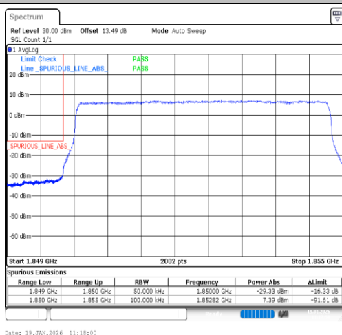
Band2-5MHz-QPSK-18625-25RB#0-PASS
