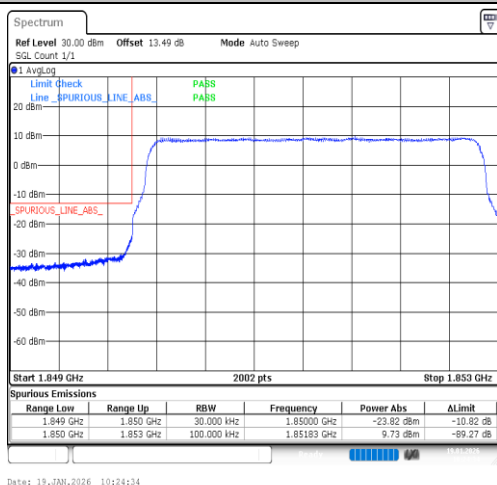
Band2-3MHz-QPSK-18615-15RB#0-PASS
