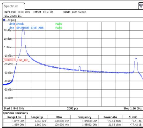
Band2-10MHz-QPSK-18650-1RB#0-PASS
