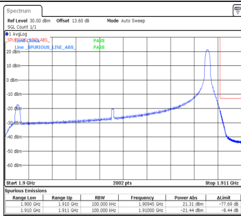
Band2-10MHz-QPSK-18650-50RB#0-PASS
