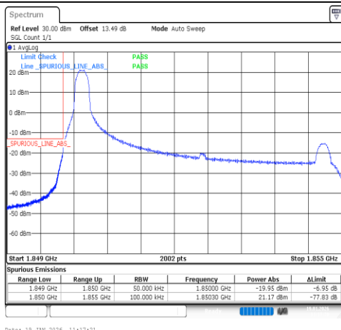
Band2-5MHz-QPSK-18625-1RB#0-PASS
