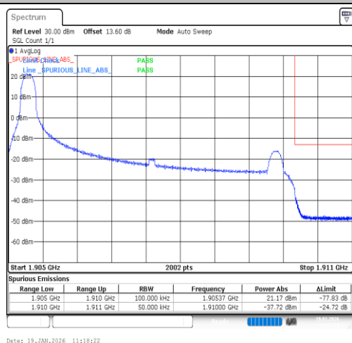
Band2-5MHz-QPSK-19175-1RB#0-PASS
