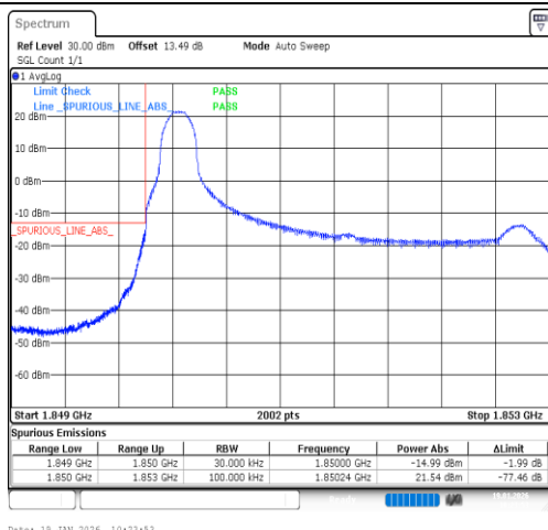
Band2-3MHz-QPSK-18615-1RB#0-PASS
