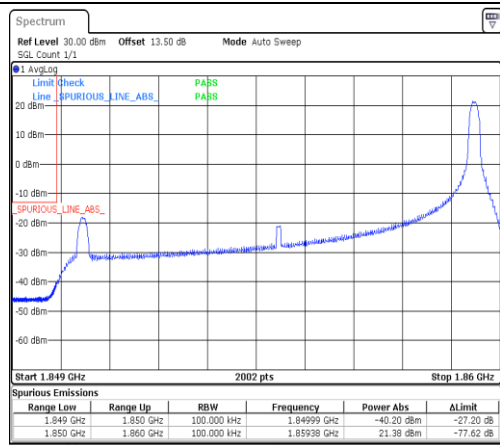
Band2-10MHz-QPSK-18650-1RB#49-PASS
