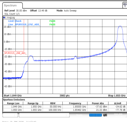
Band2-5MHz-QPSK-18625-1RB#24-PASS
