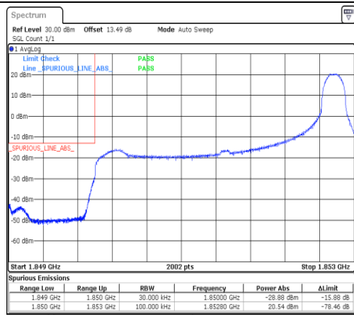
Band2-3MHz-16QAM-18615-1RB#14-PASS
