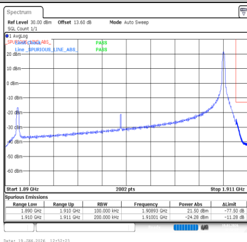
Band2-20MHz-QPSK-19100-1RB#99-PASS
