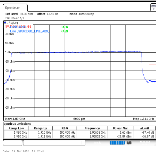
Band2-20MHz-QPSK-19100-100RB#0-PASS
