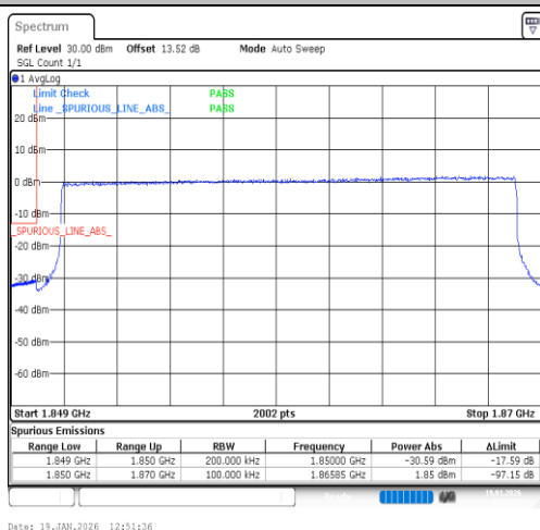
Band2-20MHz-QPSK-18700-100RB#0-PASS
