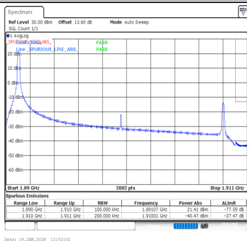
Band2-20MHz-QPSK-19100-1RB#0-PASS
