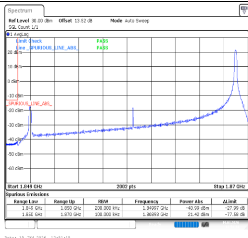
Band2-20MHz-QPSK-18700-1RB#99-PASS
