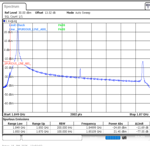
Band2-20MHz-QPSK-18700-1RB#0-PASS
