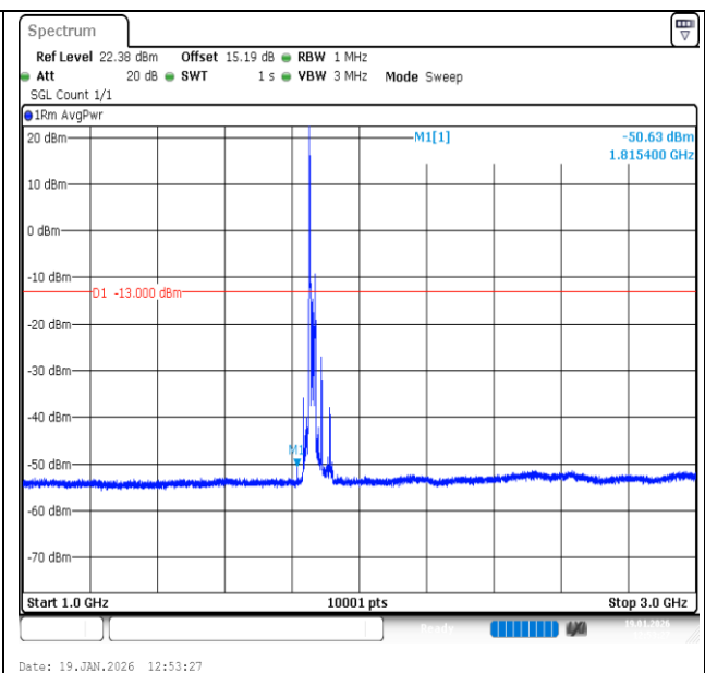
Band2-20MHz-QPSK-18700-1RB#0-1000~3000-PASS
