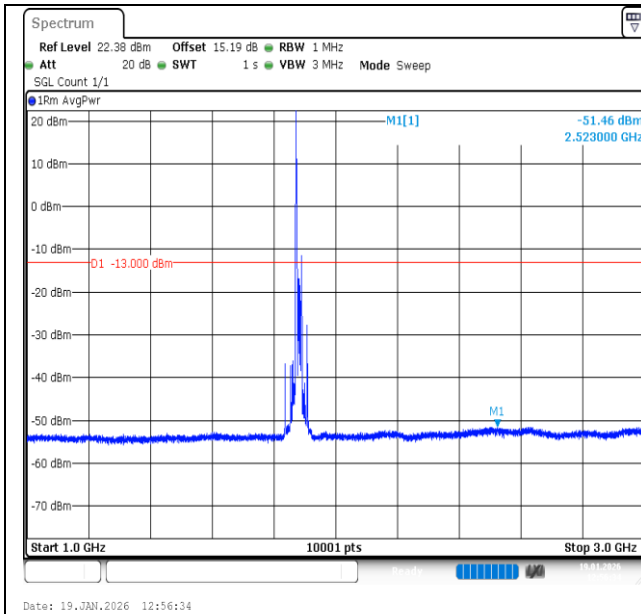
Band2-20MHz-QPSK-18900-1RB#0-1000~3000-PASS
