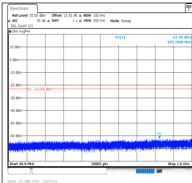
Band2-20MHz-QPSK-18700-1RB#0-30~1000-PASS
