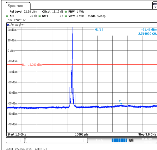
Band2-20MHz-QPSK-18700-1RB#99-1000~3000-PASS
