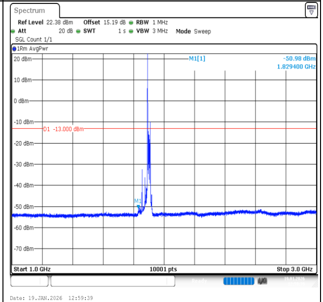
Band2-20MHz-QPSK-19100-1RB#0-1000~3000-PASS
