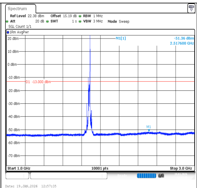
Band2-20MHz-QPSK-18900-1RB#99-1000~3000-PASS
