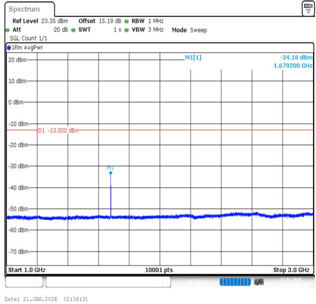
Band26 (824-849)-10MHz-QPSK-26990-1RB#0-1000~3000-PASS
