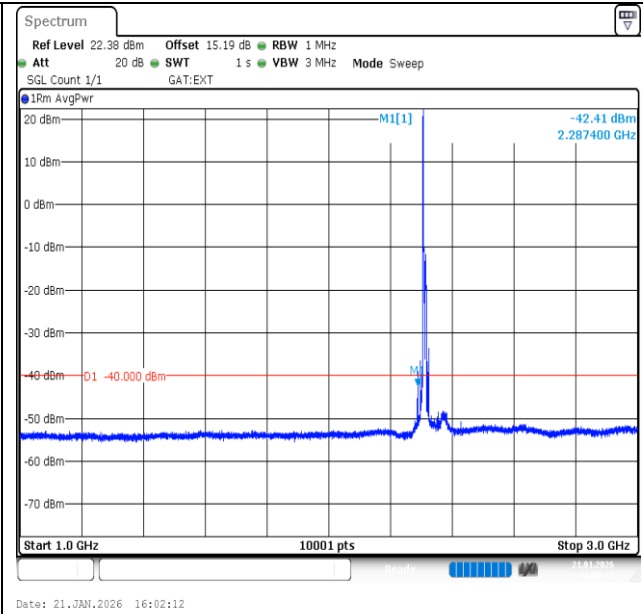
Band40 (2305-2315)-10MHz-QPSK-38750-1RB#0-1000~3000-PASS
