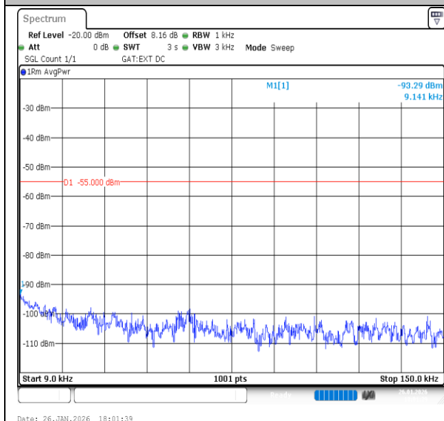
Band41-10MHz-QPSK-41540-50RB#0-0.009~0.15-PASS
