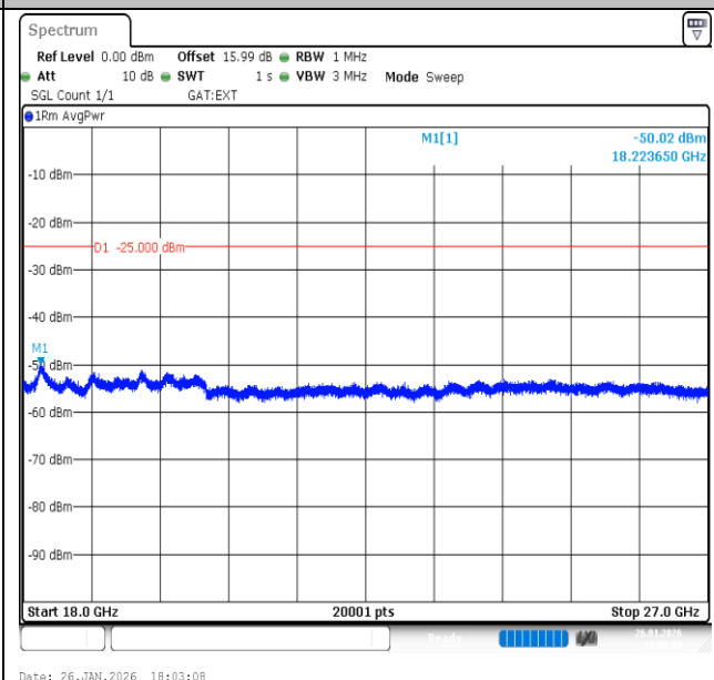
Band41-10MHz-QPSK-41540-50RB#0-18000~27000-PASS
