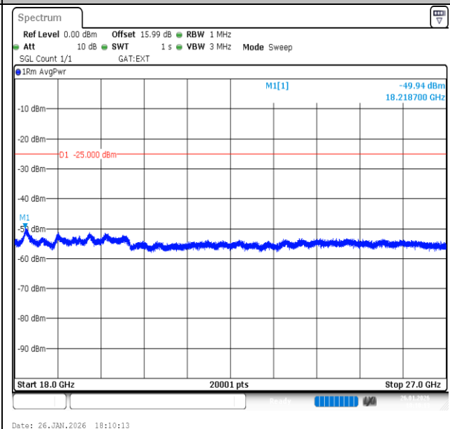
Band41-15MHz-QPSK-39725-1RB#0-18000~27000-PASS
