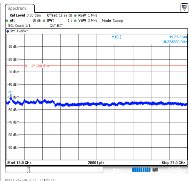
Band41-15MHz-16QAM-41515-1RB#0-18000~27000-PASS
