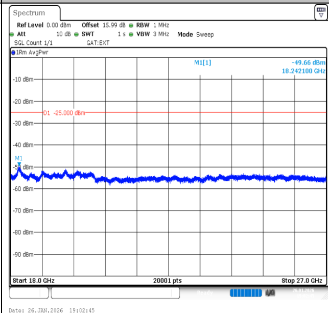
Band41-15MHz-16QAM-41515-1RB#74-18000~27000-PASS
