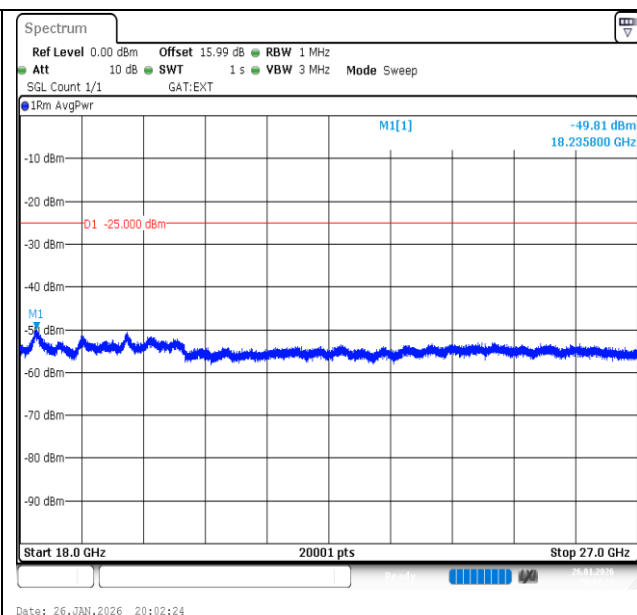
Band41-20MHz-QPSK-41490-1RB#99-18000~27000-PASS
