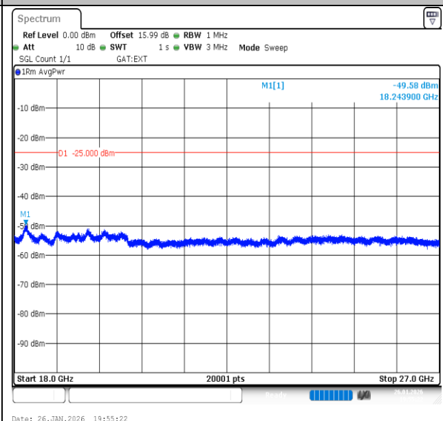
Band41-20MHz-QPSK-41490-1RB#0-18000~27000-PASS
