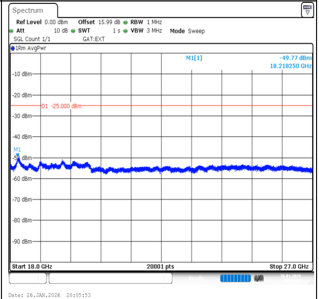
Band41-20MHz-16QAM-41490-1RB#99-18000~27000-PASS
