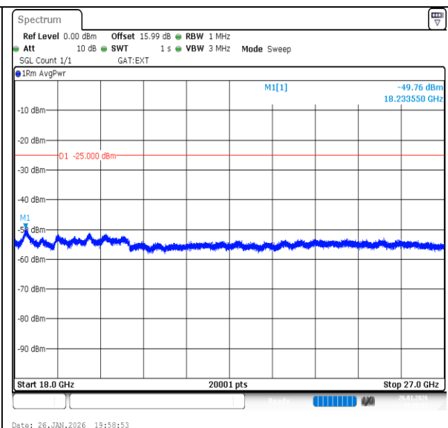
Band41-20MHz-16QAM-41490-1RB#0-18000~27000-PASS
