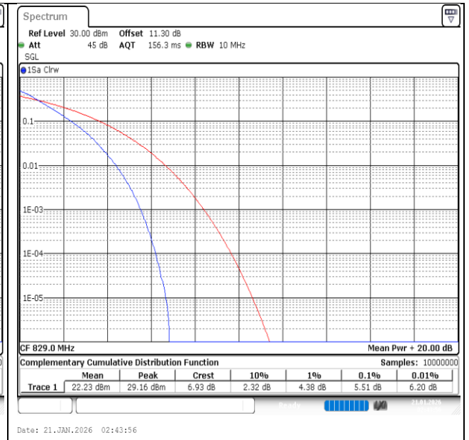
Band26(824-849)-10MHz-QPSK-26840-50RB#0-PASS
