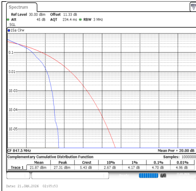
Band26(824-849)-3MHz-QPSK-27025-1RB#0-PASS
