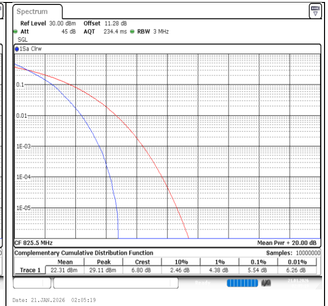
Band26(824-849)-3MHz-QPSK-26805-15RB#0-PASS
