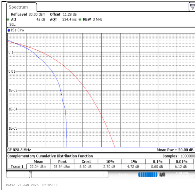
Band26(824-849)-3MHz-QPSK-26805-1RB#0-PASS
