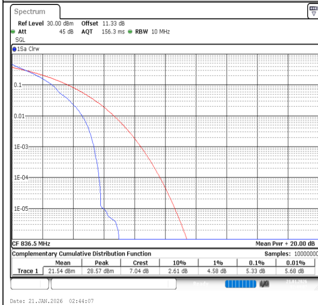
Band26(824-849)-10MHz-QPSK-26915-1RB#0-PASS
