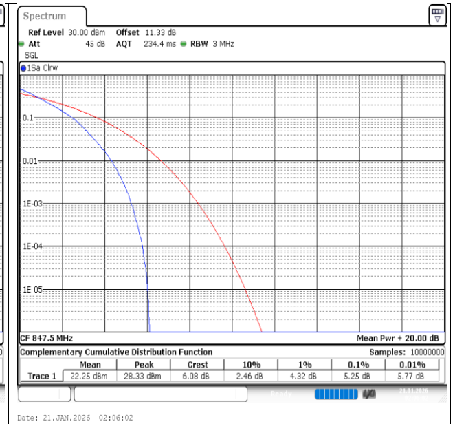
Band26(824-849)-3MHz-QPSK-27025-15RB#0-PASS
