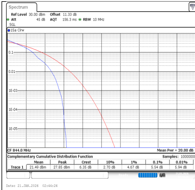
Band26(824-849)-10MHz-QPSK-26990-1RB#0-PASS
