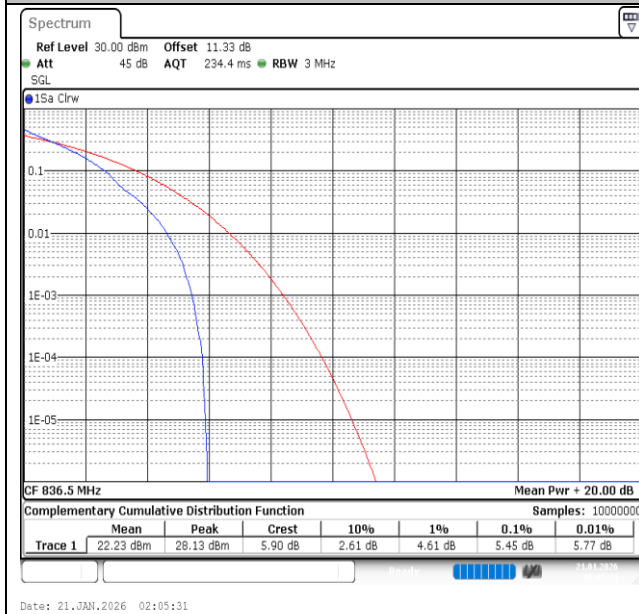
Band26(824-849)-3MHz-QPSK-26915-1RB#0-PASS
