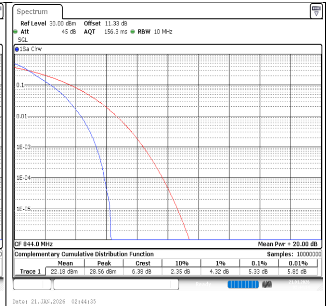
Band26(824-849)-10MHz-QPSK-26990-50RB#0-PASS
