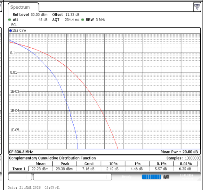
Band26(824-849)-3MHz-QPSK-26915-15RB#0-PASS
