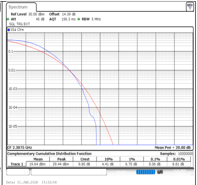
Band40(2305-2315)-5MHz-QPSK-38725-25RB#0-PASS
