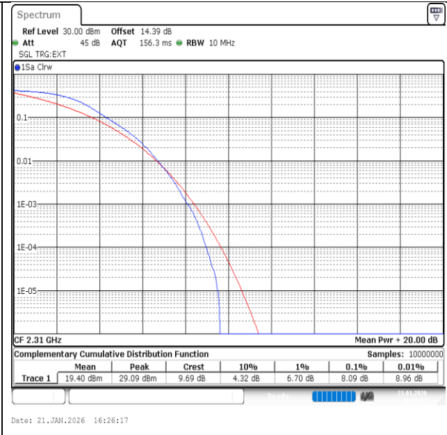
Band40(2305-2315)-10MHz-QPSK-38750-50RB#0-PASS
