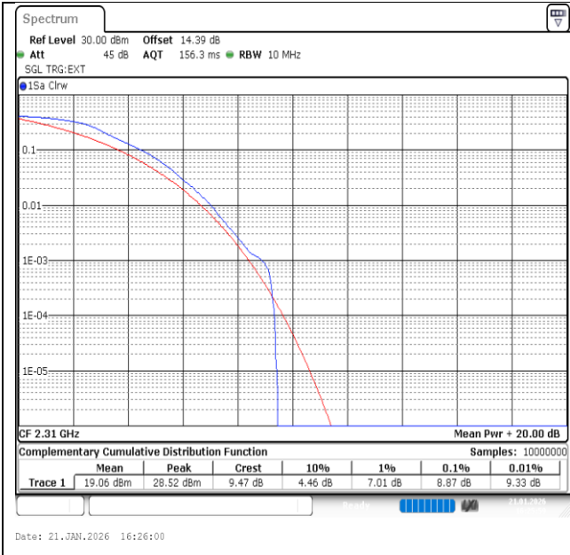
Band40(2305-2315)-10MHz-QPSK-38750-1RB#0-PASS
