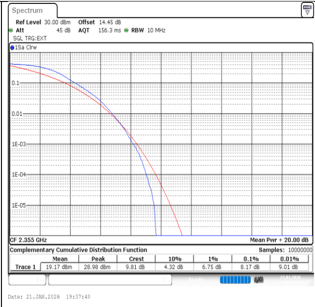
Band40(2350-2360)-10MHz-QPSK-39200-50RB#0-PASS
