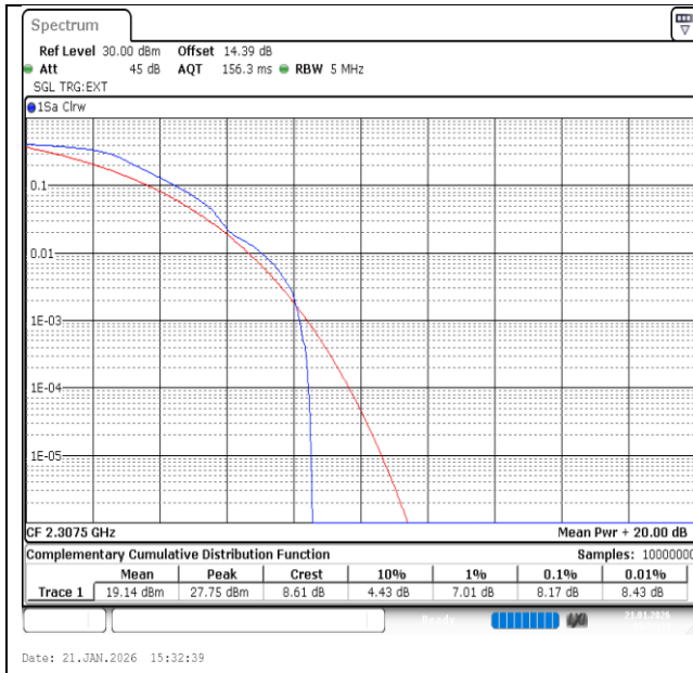
Band40(2305-2315)-5MHz-QPSK-38725-1RB#0-PASS
