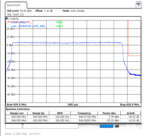
Band26(824-849)-10MHz-QPSK-26990-50RB#0-P ASS
