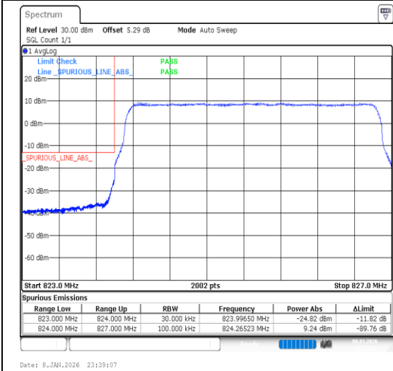
Band26(824-849)-3MHz-QPSK-26805-15RB#0-PA SS
