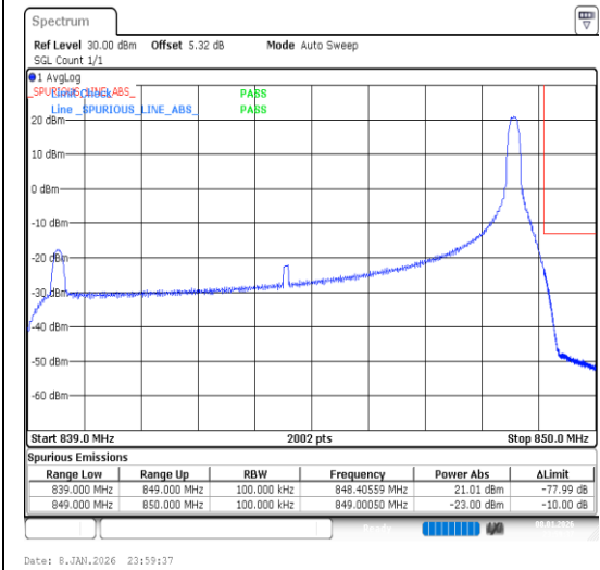
Band26(824-849)-10MHz-QPSK-26990-1RB#49-P ASS
