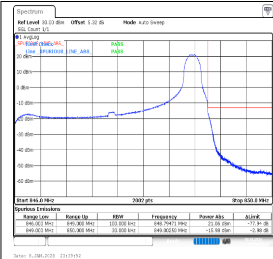
Band26(824-849)-3MHz-QPSK-27025-1RB#14-PA SS
