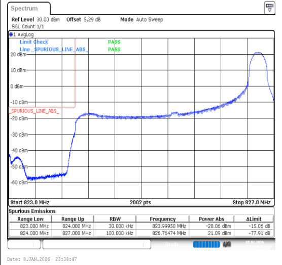
Band26(824-849)-3MHz-QPSK-26805-1RB#14-P ASS
