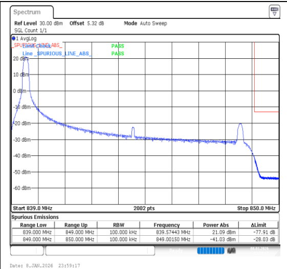
Band26(824-849)-10MHz-QPSK-26990-1RB#0-P ASS
