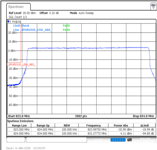
Band26(824-849)-10MHz-QPSK-26840-50RB#0-P ASS
