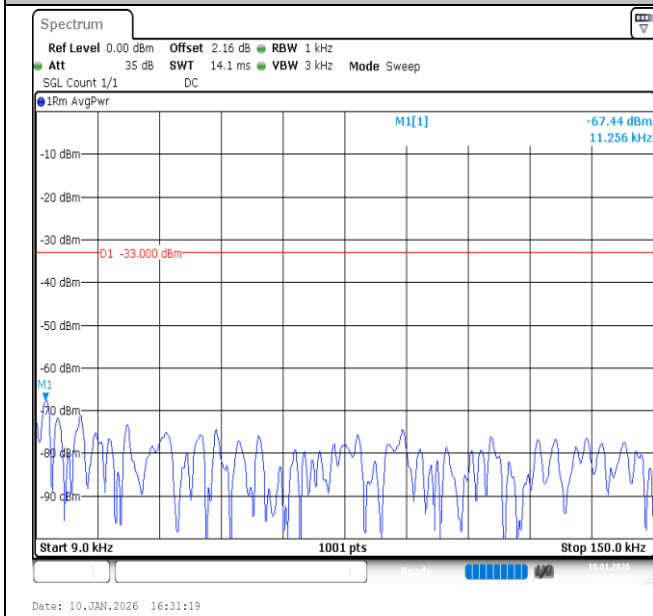
Band26 (824-849)-10MHz-QPSK-26840-50RB#0-0.009~0.15-PASS
