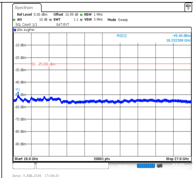
Band41-10MHz-QPSK-41540-50RB#0-18000~27000-PASS
