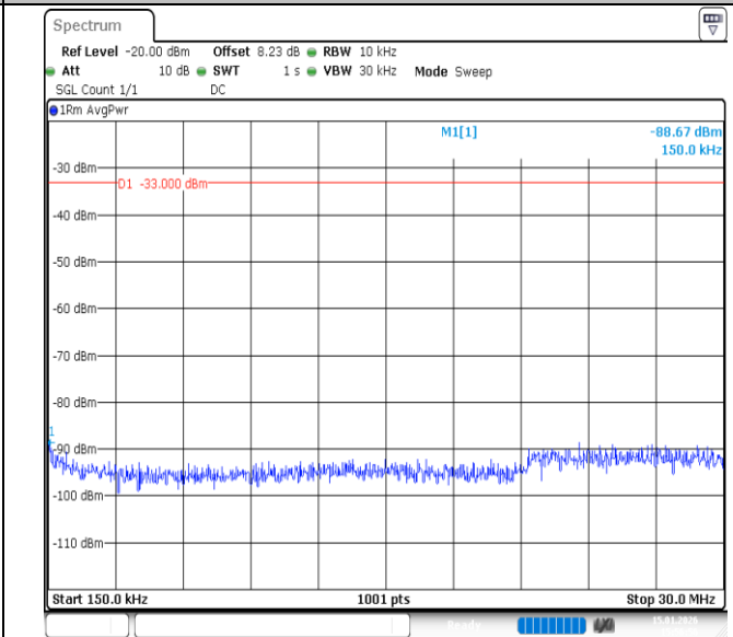
Band66-20MHz-QPSK-132572-1RB#99-3000-20000-PASS
