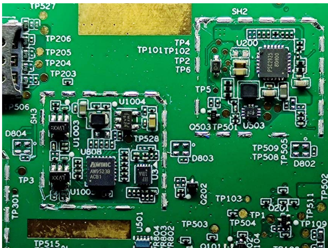
WWAN Module A Main Antenna
