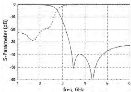
RFLPF16081G8DC8Q1C
