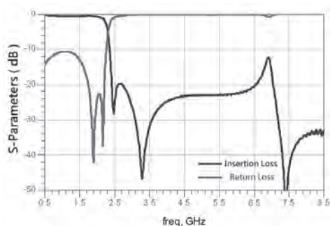
RFLPF16081G8DC8Q1C
