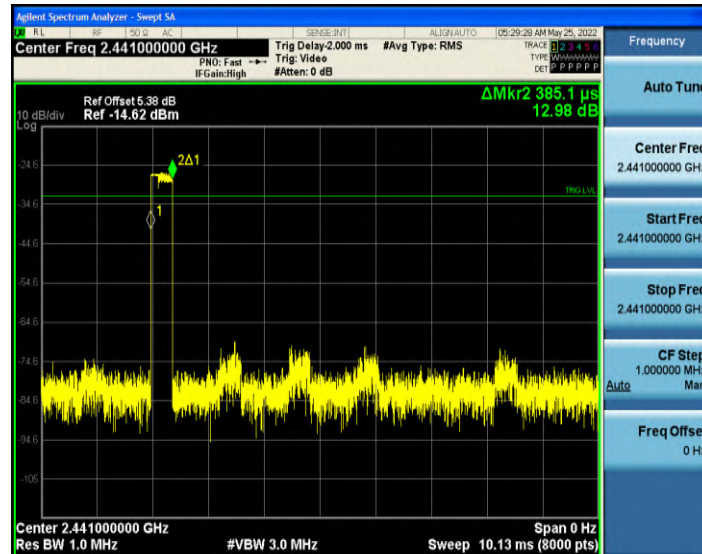
2DH3_Ant1_Hop
