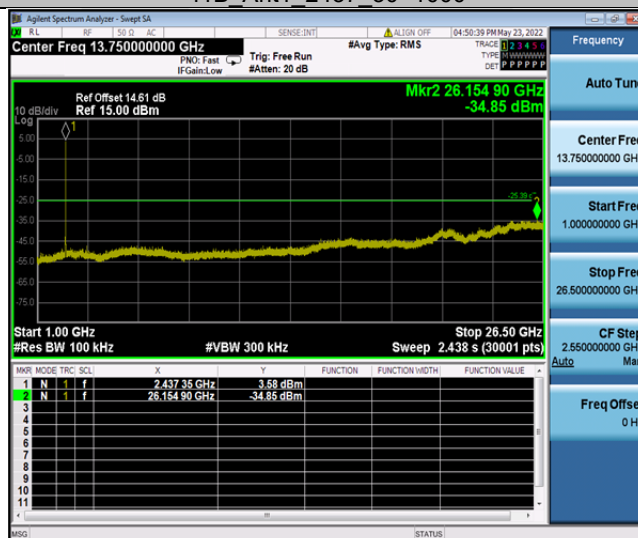
11B_Ant1_2437_1000~26500
