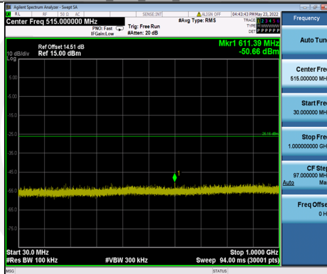
11B_Ant1_2412_30~1000
