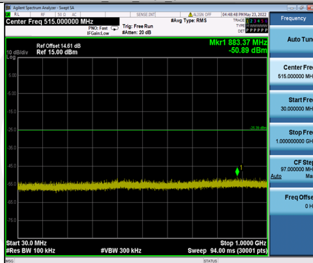
11B_Ant1_2437_30~1000
