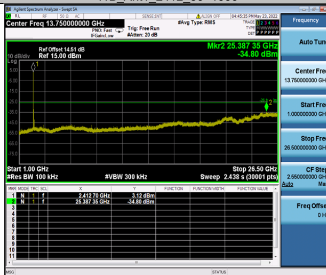
11B_Ant1_2412_1000~26500
