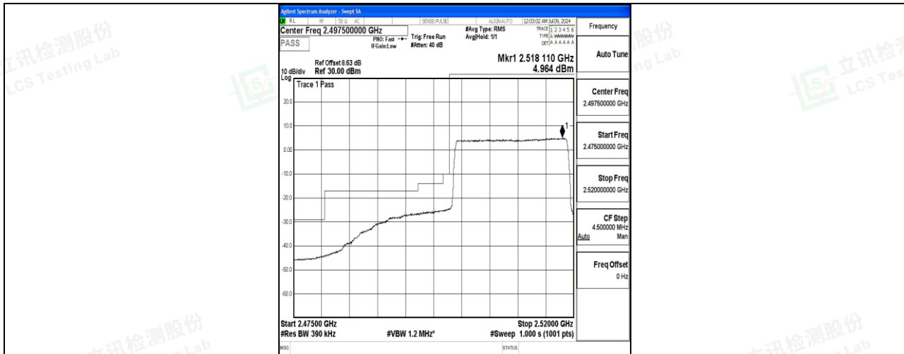
Band7_20MHz_16QAM_20850_100RB#0
