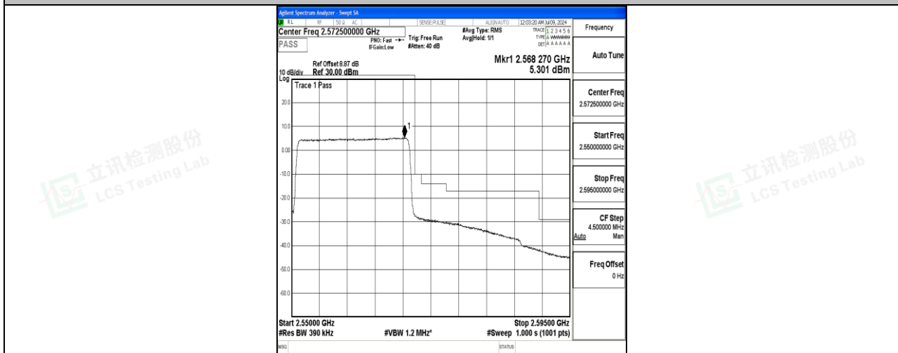
Band7_20MHz_16QAM_21350_100RB#0
