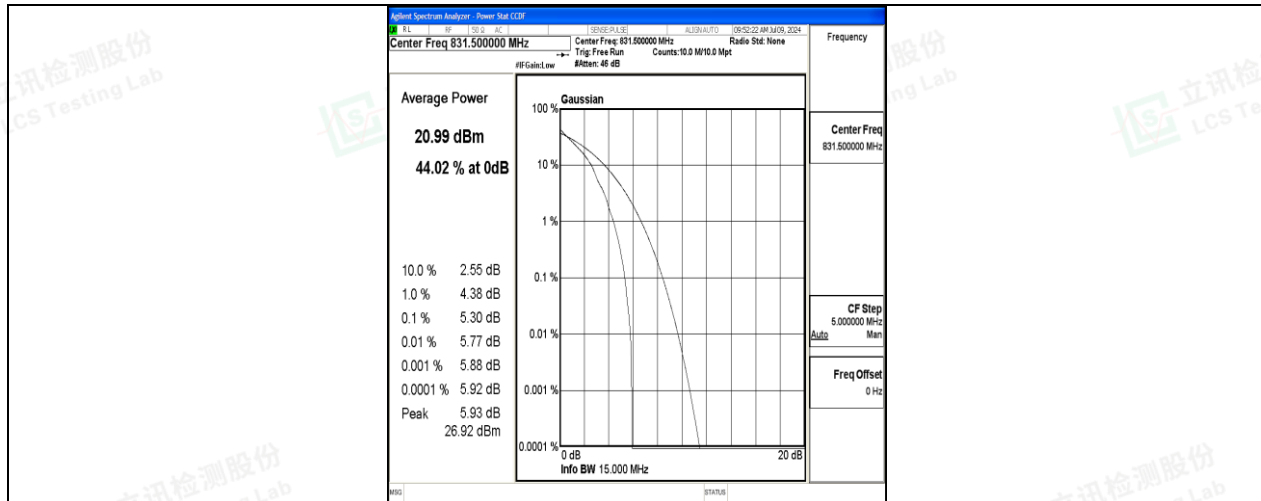
26(824-849)-15MHz-QPSK-26865-1RB#0-PASS
