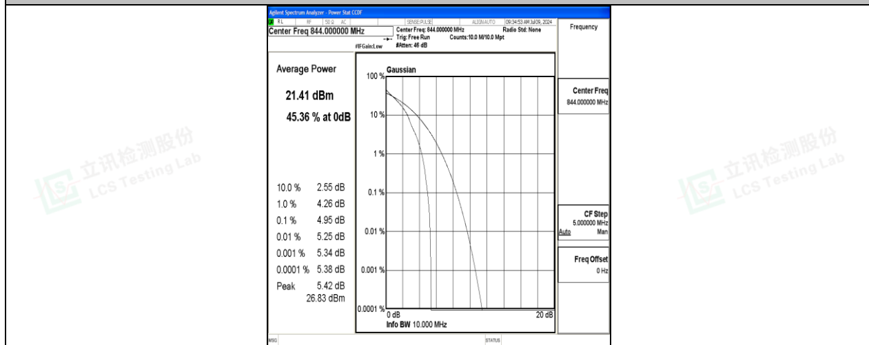
26(824-849)-10MHz-QPSK-26990-1RB#0-PASS
