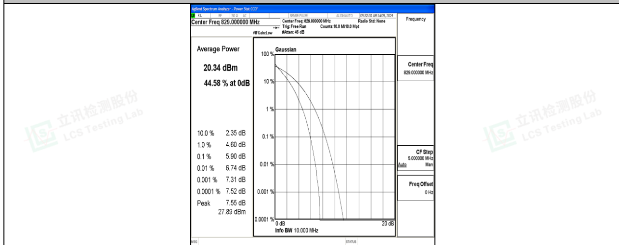
26(824-849)-10MHz-QPSK-26840-50RB#0-PASS
