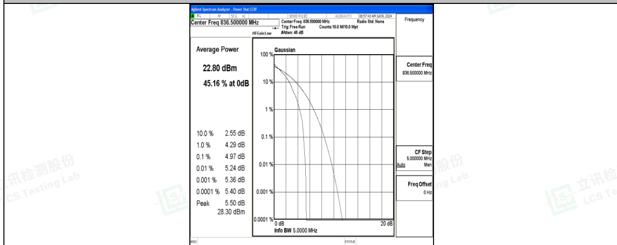
26(824-849)-3MHz-QPSK-26915-1RB#0-PASS
