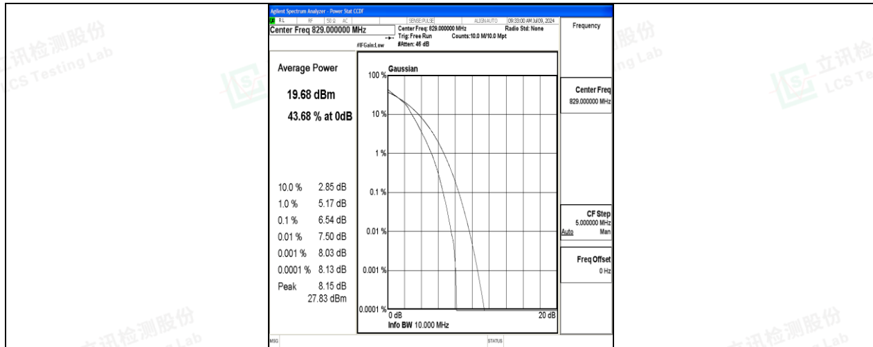
26(824-849)-10MHz-16QAM-26840-50RB#0-PASS
