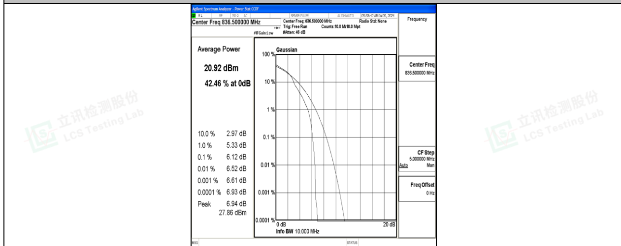
26(824-849)-10MHz-16QAM-26915-1RB#0-PASS
