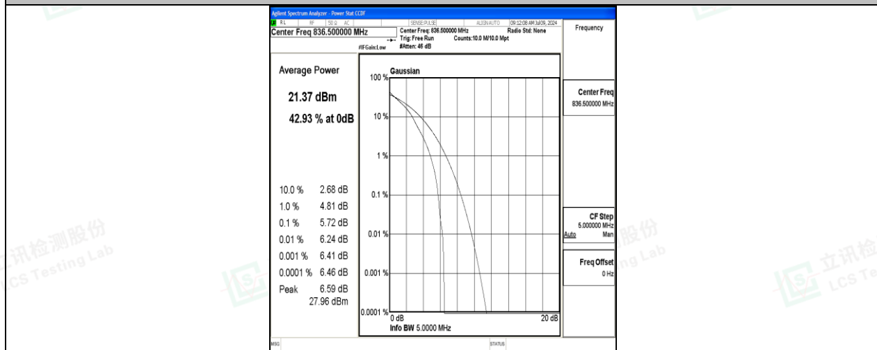
26(824-849)-5MHz-QPSK-26915-1RB#0-PASS
