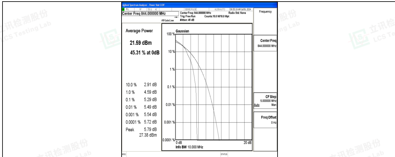
26(824-849)-10MHz-16QAM-26990-1RB#0-PASS
