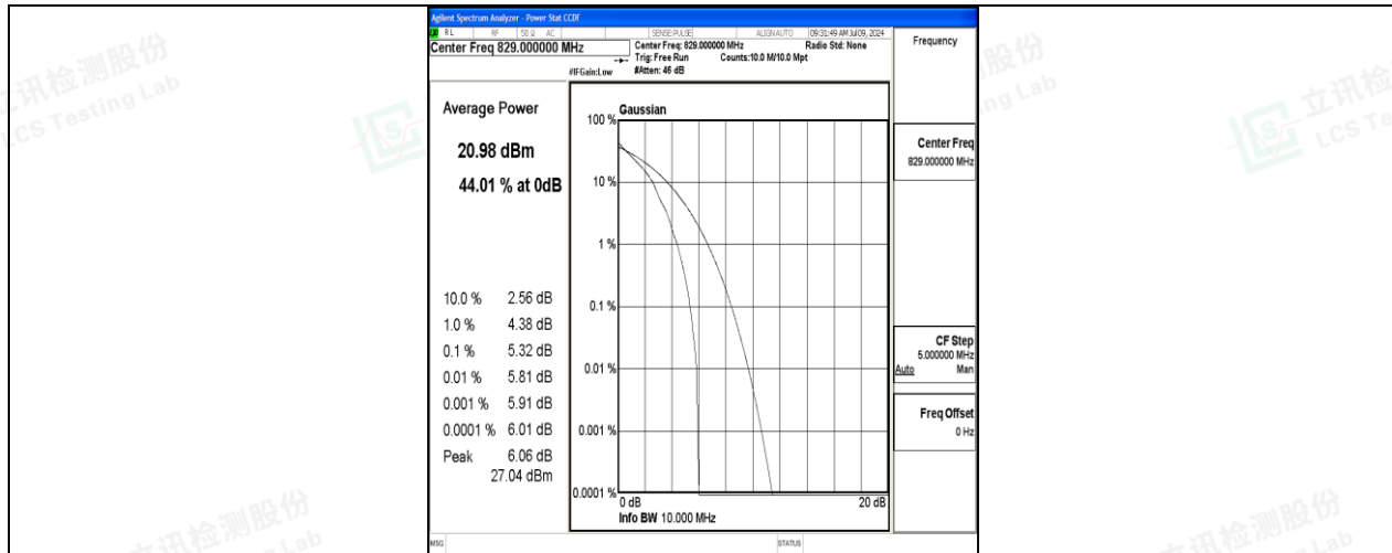
26(824-849)-10MHz-QPSK-26840-1RB#0-PASS
