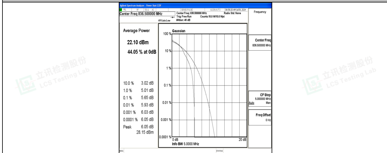
26(824-849)-3MHz-16QAM-26915-1RB#0-PASS
