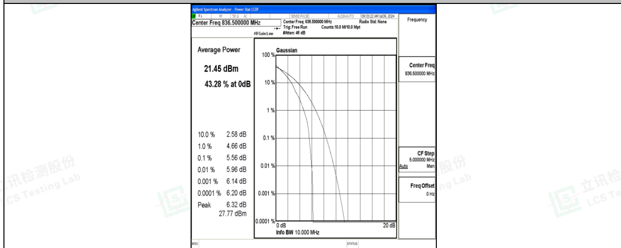
26(824-849)-10MHz-QPSK-26915-1RB#0-PASS
