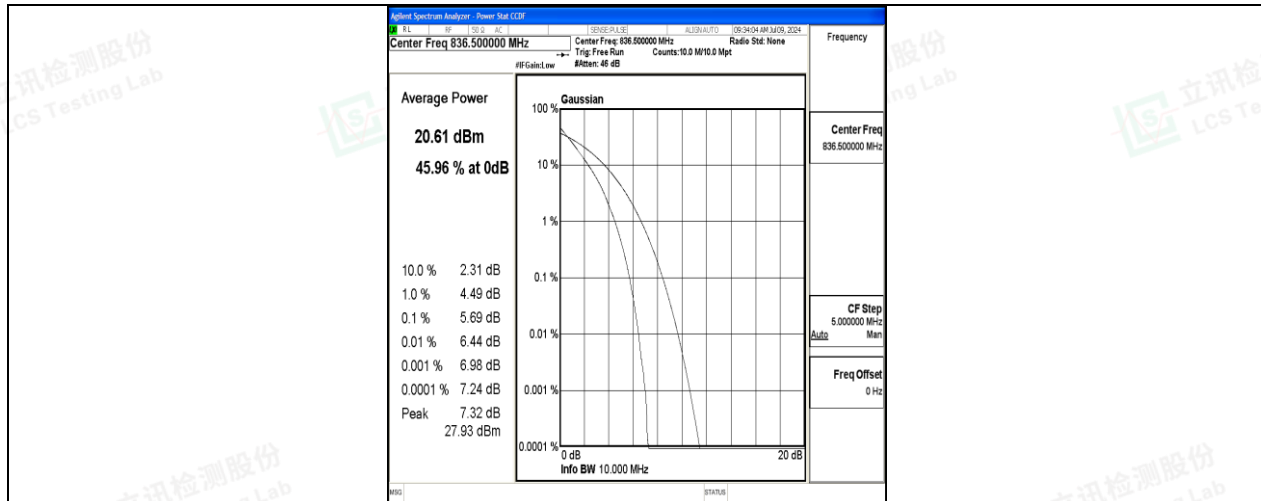
26(824-849)-10MHz-QPSK-26915-50RB#0-PASS
