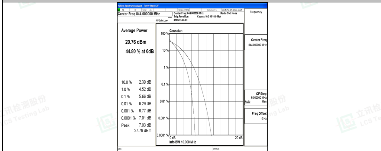
26(824-849)-10MHz-QPSK-26990-50RB#0-PASS
