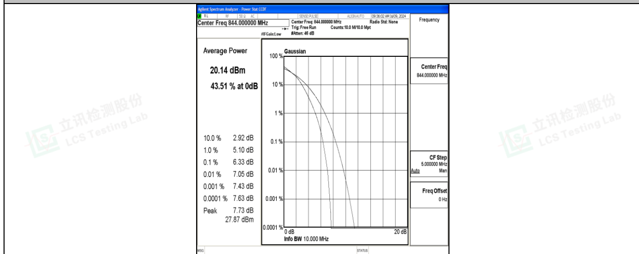
26(824-849)-10MHz-16QAM-26990-50RB#0-PASS
