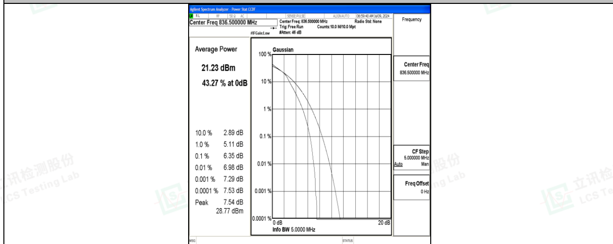
26(824-849)-3MHz-16QAM-26915-15RB#0-PASS
