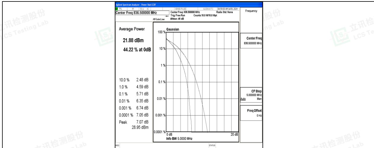
26(824-849)-3MHz-QPSK-26915-15RB#0-PASS
