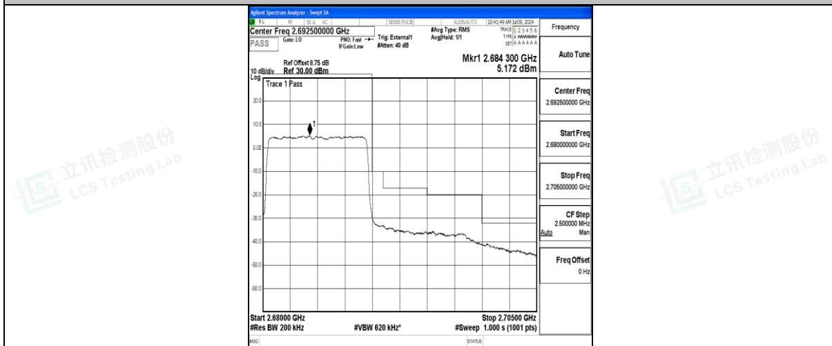
Band41_10MHz_QPSK_41540_50RB#0
