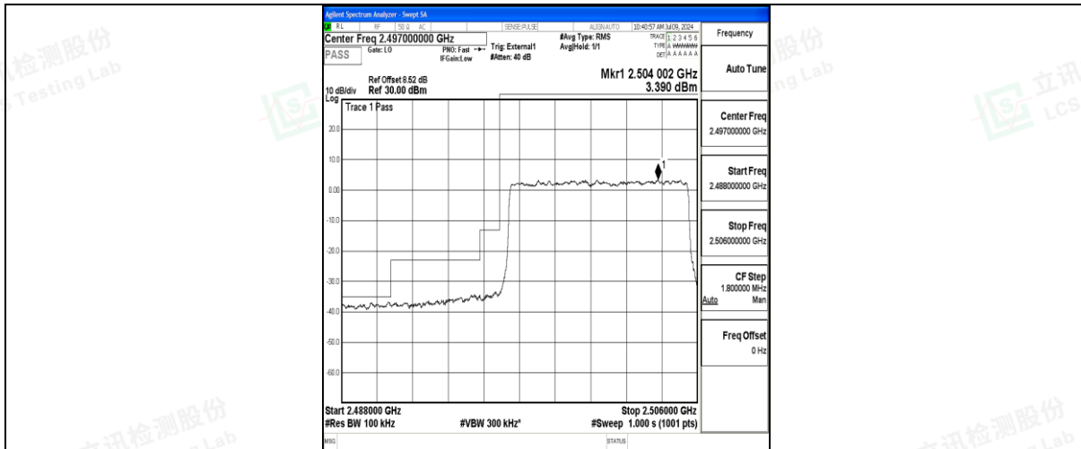
Band41_10MHz_QPSK_39700_50RB#0
