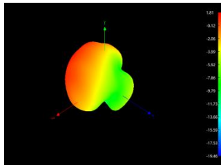
2450MHz
