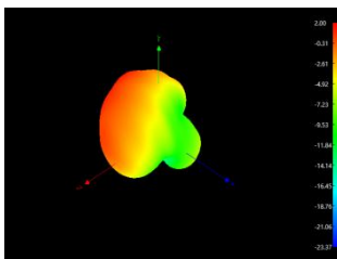
2450MHz
