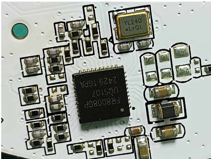
BLE radio 1
