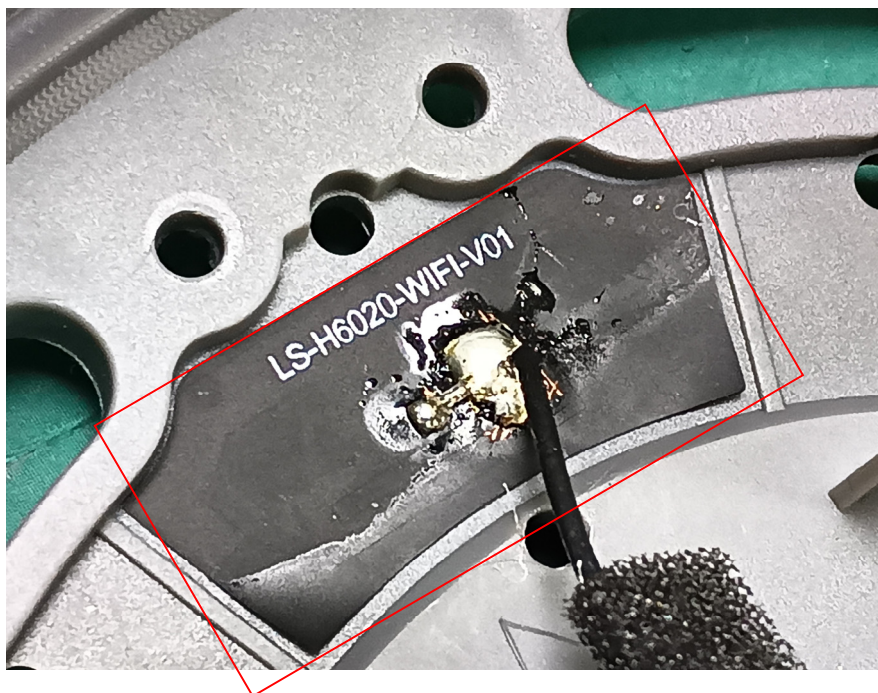
2.4G Wi-Fi ANT & BLE ANT(Radio2)
