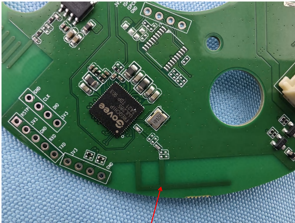
BLE-ANT
