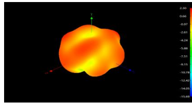
2400MHz
