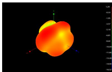
2400MHz
