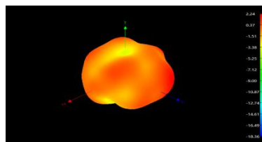
2500MHz
