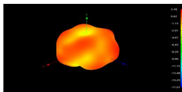
2450MHz
