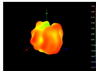
2450MHz
