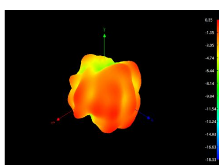
2500MHz
