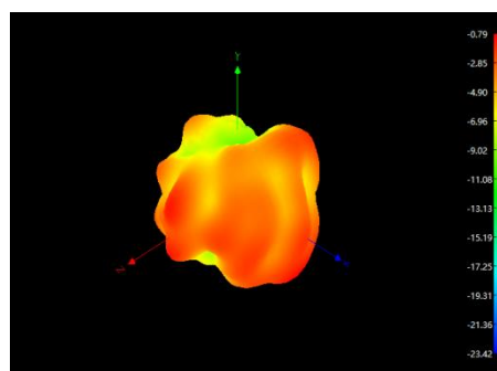
2500MHz
