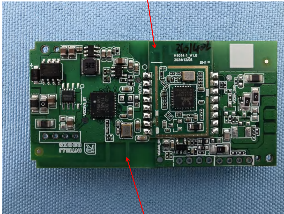
BLE-ANT
