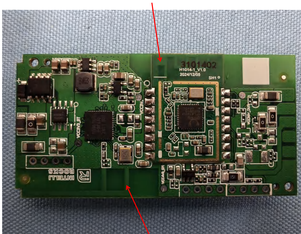
BLE-ANT
