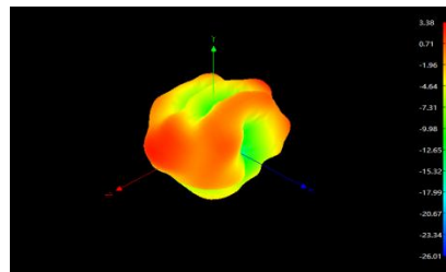
2500MHz
