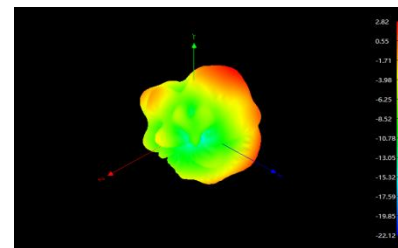
2450MHz
