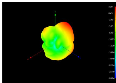
2400MHz
