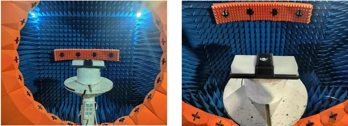
3. DUT Setup Photo
