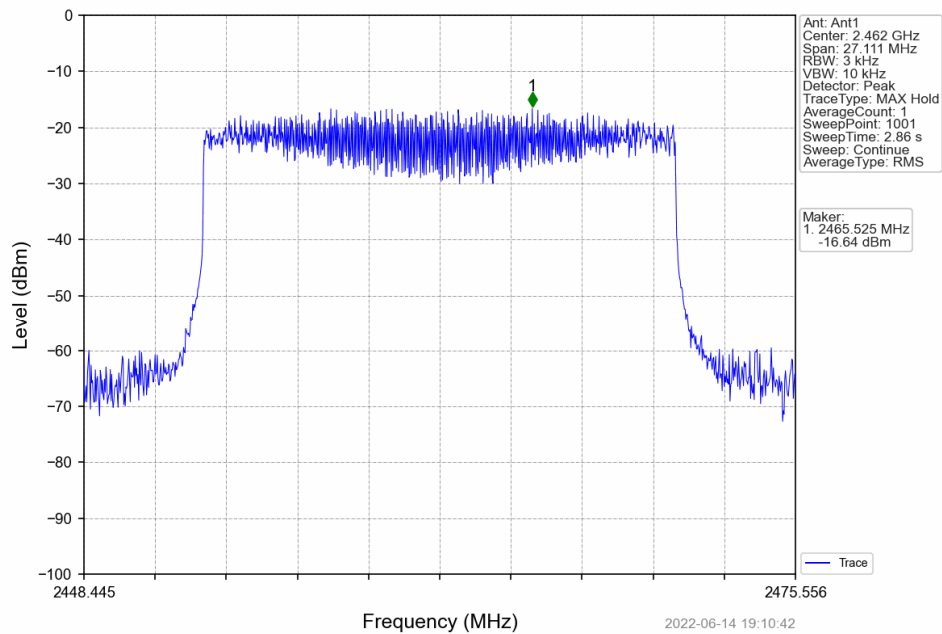
QPSK2_HCH_2462MHz_Ant1_NTNV
