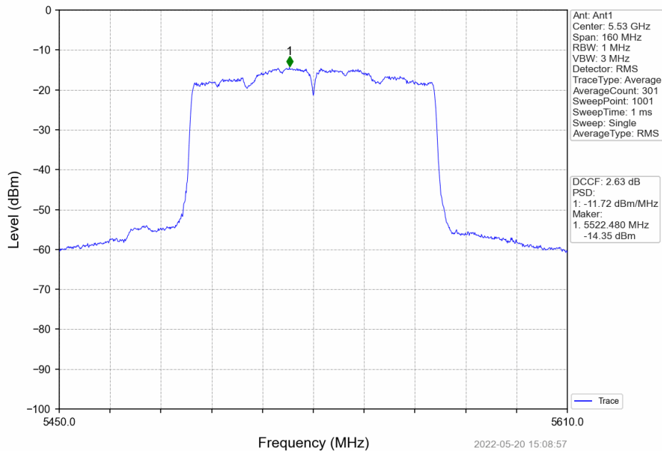
802.11ac(VHT80)_LCH_5530MHz_Ant1_NTNV
