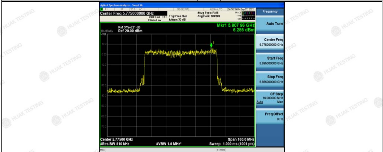
High 802.11ax(HT80)
