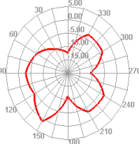
2450.000MHz E2
