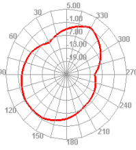
2450.000MHz H
