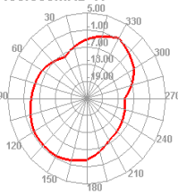
2400.000MHz E2
