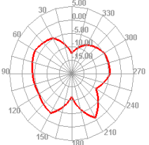
2450.000MHz E1
