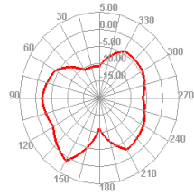
2500.000MHz E2
