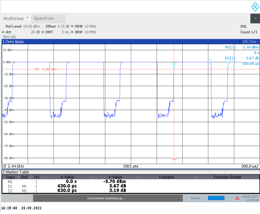
BLE_1M_2440MHz
