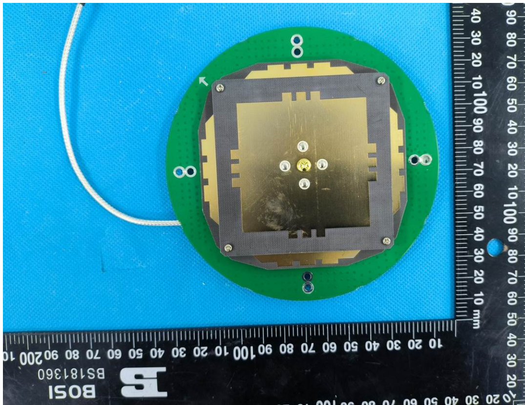
GPS Antenna
