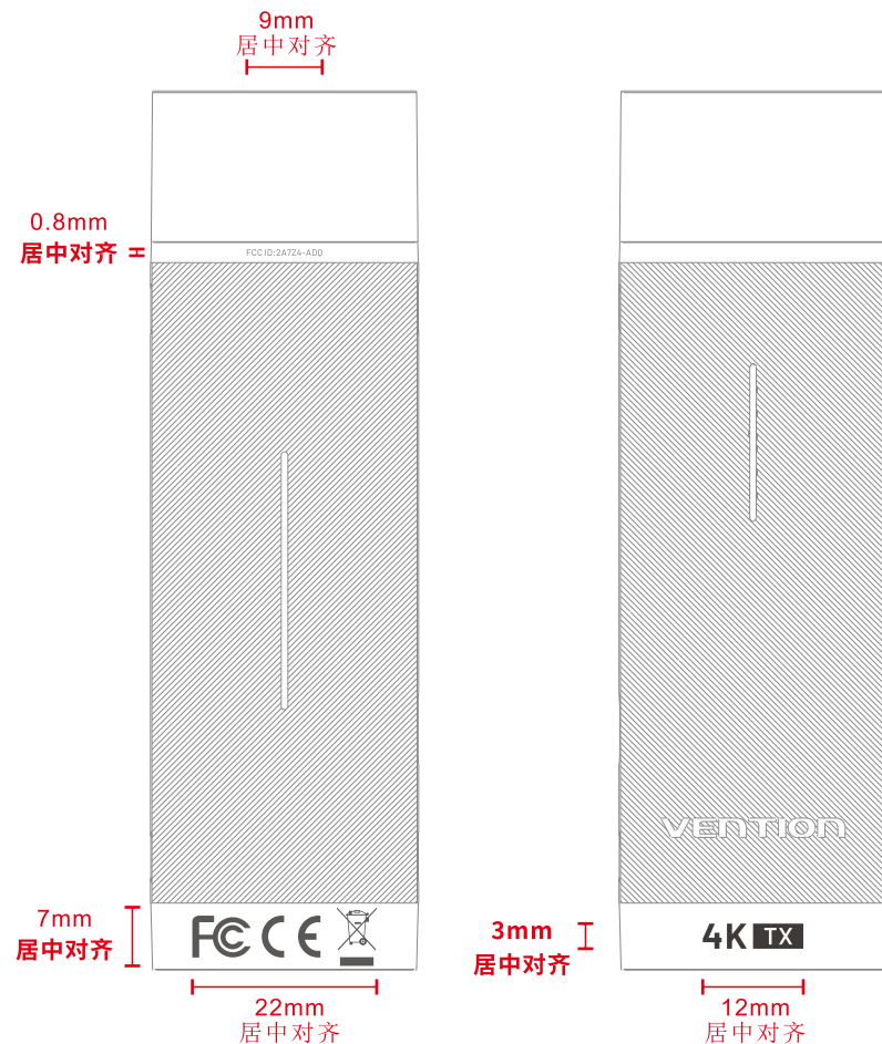
发射端背面
