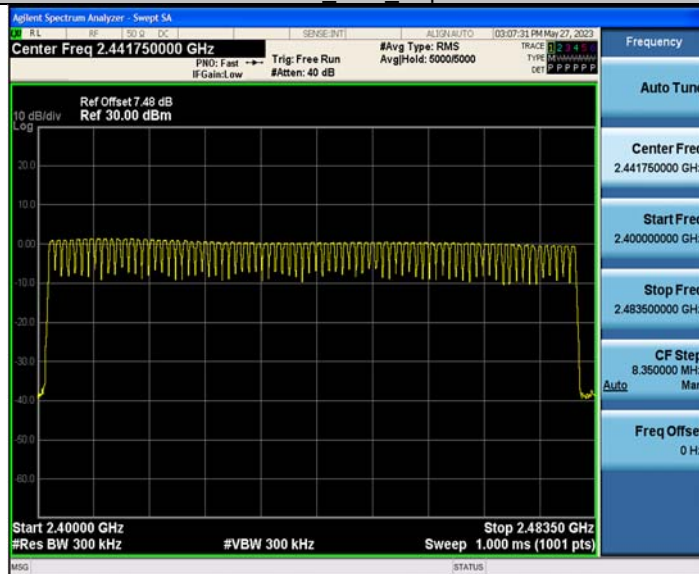
DH5_Ant2_Hop
