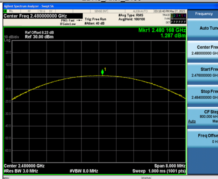
2DH5_Ant2_2480
