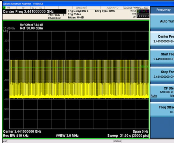
DH1_Ant2_Hop
