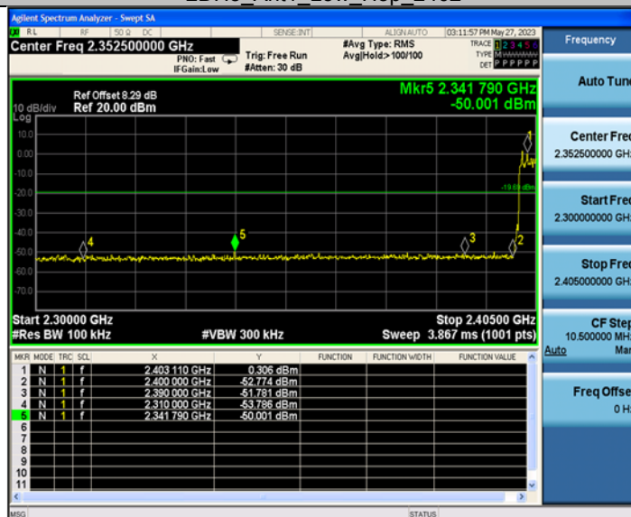
2DH5_Ant2_Low_Hop_2402
